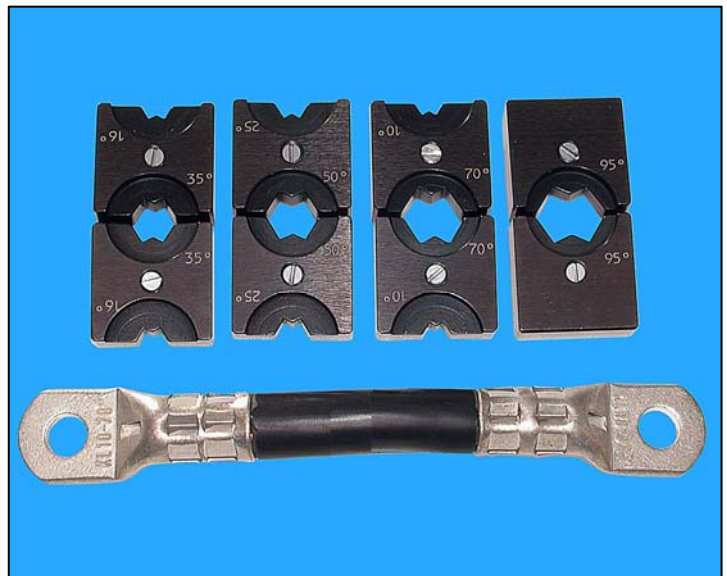
Doppel-W-Crimp-Set für Rohrkabelschuhe (10 - 95 mm 2 ) Double-W-Crimp-Set for Copper-Tube Terminals (10 - 95 mm 2 ) Set de sertissage double-W pour des cosses tubulaires (10 - 95 mm 2 ) Heavy-Duty-Gesenkaufnahme mit DW-Crimp-Gesenk 120mm 2 Heavy-Duty-Die-Holder with double-W-die 120mm 2 Heavy-Duty-adaptateur avec matrice double-W de 120mm 2
